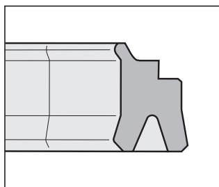
1PL Dicht-Abstreifer für verdreh- gesicherte Zylinder Seal Wiper for rotation pro- tected cylinders
