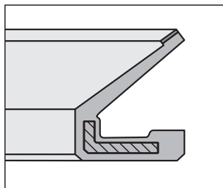
VA7-C mit reibungsoptimierter Dichtlippe aus PTFE with friction optimized sealing lip of PTFE
