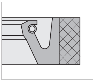
WG5-A Standardausführung Standard version
