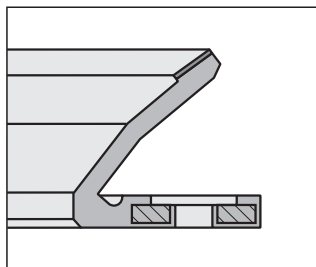
VA8-C mit reibungsoptimierter Dichtlippe aus PTFE with friction optimized sealing lip of PTFE
