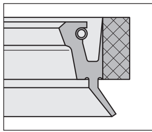
WG4 Standardausführung Standard version
