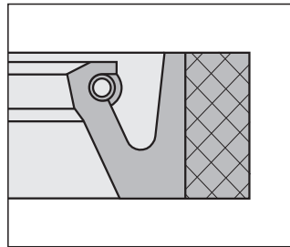
WG5-B mit vergossener Feder with covered spring
