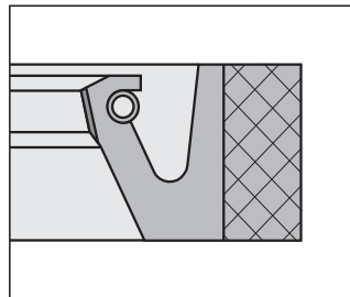
WG5-C mit reibungsoptimierter Dichtlippe with friction optimised sealing lip
