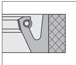
WG5-D mit vergossener Feder und reibungsoptimierter Dichtlippe with covered spring and friction optimised sealing lip
